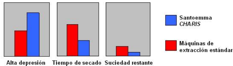
Sistema de limpieza de inyección-extracción con cepillos contragiratorios
